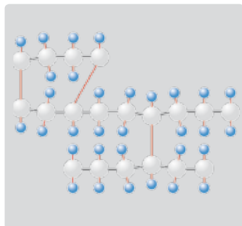
Vernette moleculaire structuur van de robuuste Uponor PE-Xa installatieleidingen
